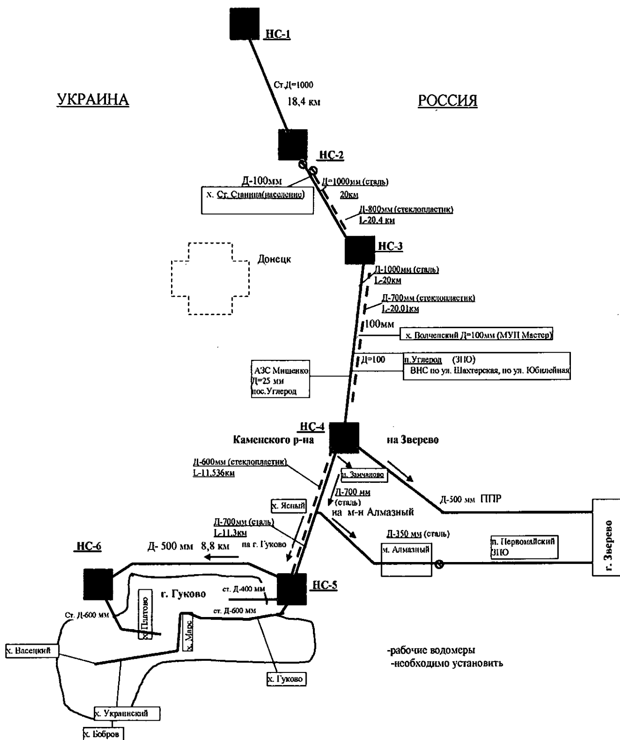
Рисунок 1.1.4.3. Принципиальная схема группового Гундорово-Гуковского водопровода
